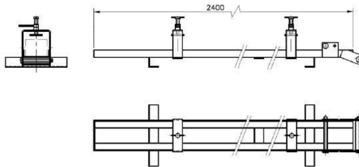
SUPORE PARA CRUZETA
