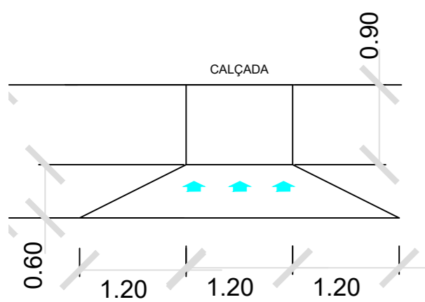
DETALHE - RAMPA DE ACESSIBILIDADE
